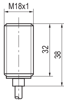
Габаритный чертеж
